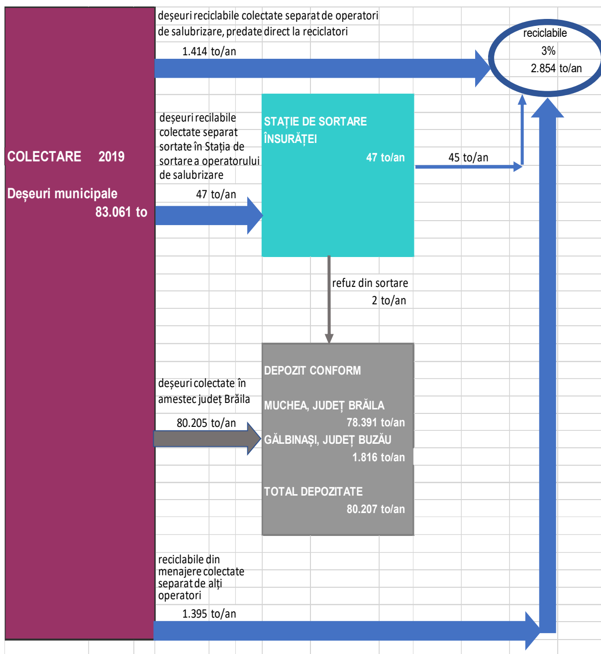
Figura 4.11. Schema fluxului de deșeuri municipale pentru anul de referință 2019
