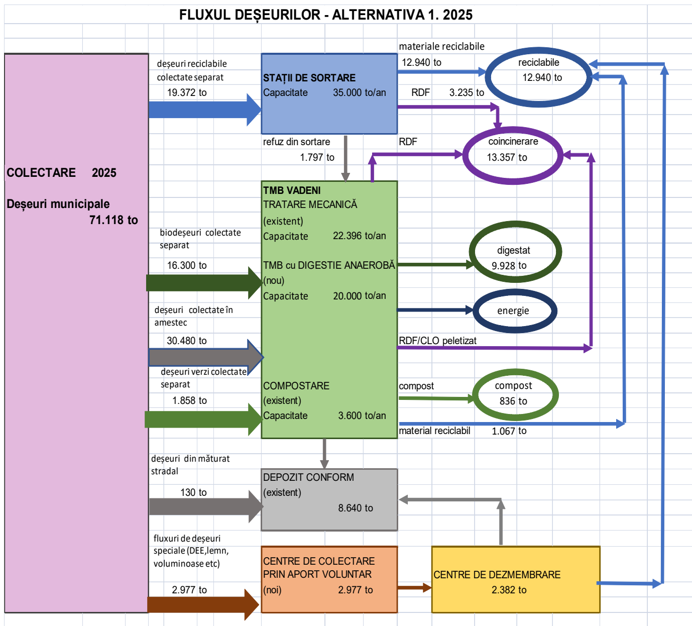
Figura 8.1. Fluxul deșeurilor. Alternativa selectată - 2025
